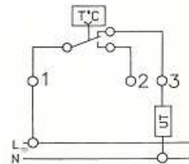
Схема переключения
