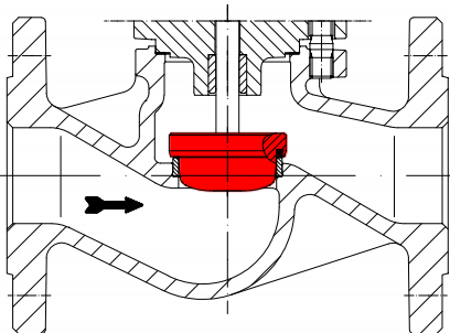
Параболический затвор с мягким уплотнением из тефлона и с направляющей штока
