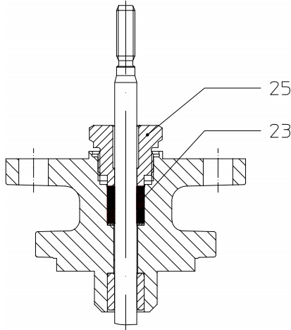
Уплотнение из тефлона/из чистого графита
