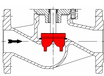
Шлицевой затвор с направляющей штока и головки
