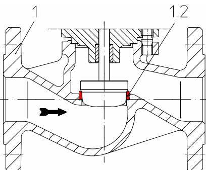
Корпус с запрессованным седлом (GG-25, GGG-40.3)
