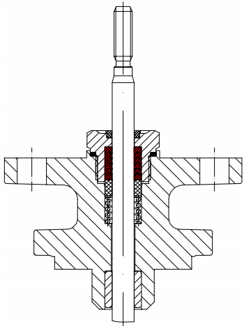
Подпружиненное уплотнение с шевронным тефлоновым кольцом
