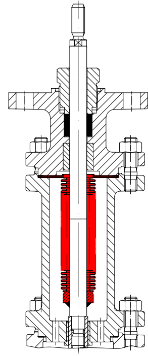
Сильфонное уплотнение с защитным корпусом
