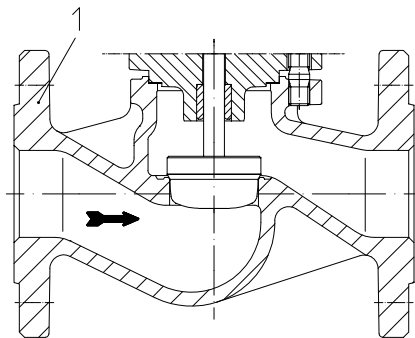
Корпус с седлом, выполненным механической обработкой (1.4408)
