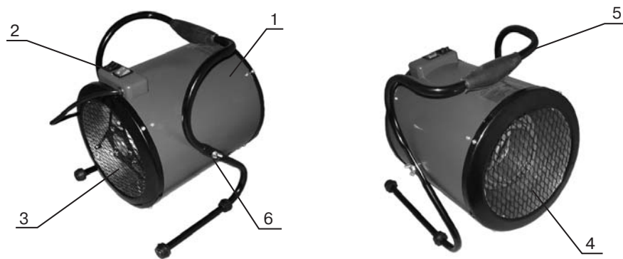
1 – кожух наружный; 2 – блок управления; 3 – входная решетка; 4 – выходная решетка; 5 – подставка; 6 – гайка.
