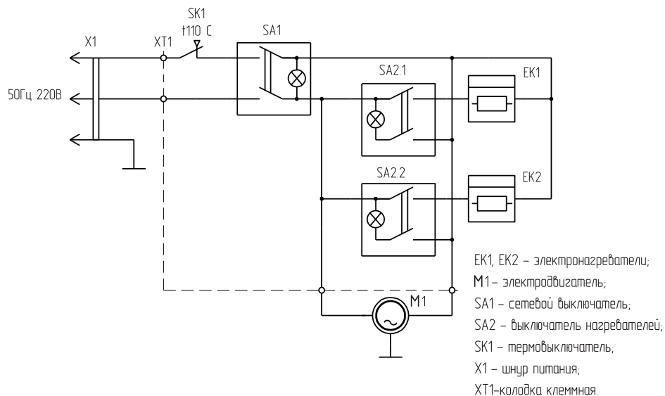
Рис. 1. Схема электрическая
